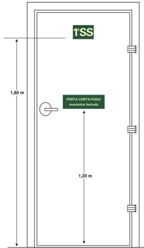
Figura 2 - Sinalização de porta corta-fogo (vista do hall)
